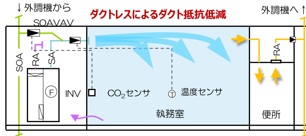
空調システム図
