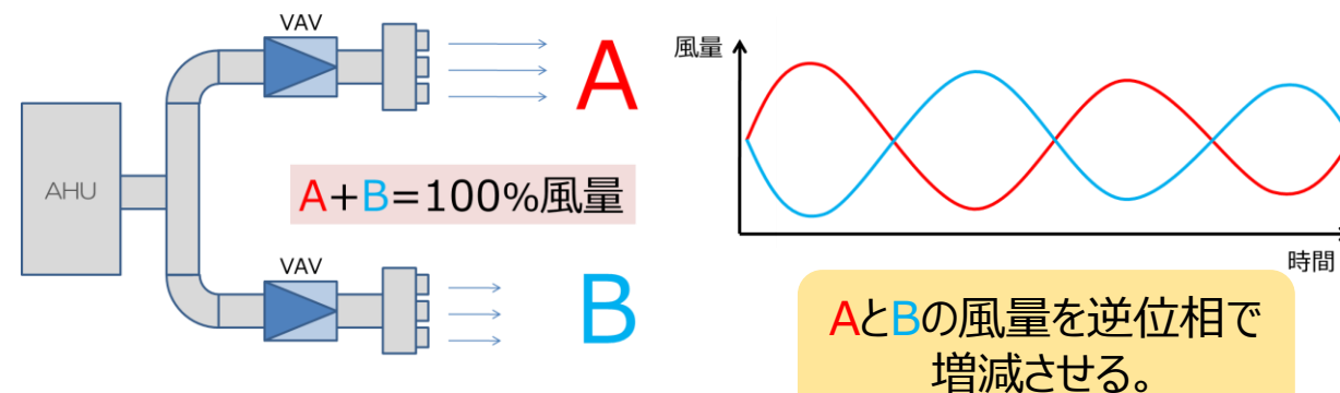
ゆらぎ制御による風の変化
